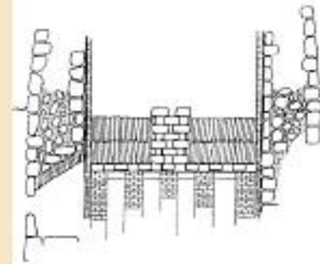
esquema do encañado do forno
